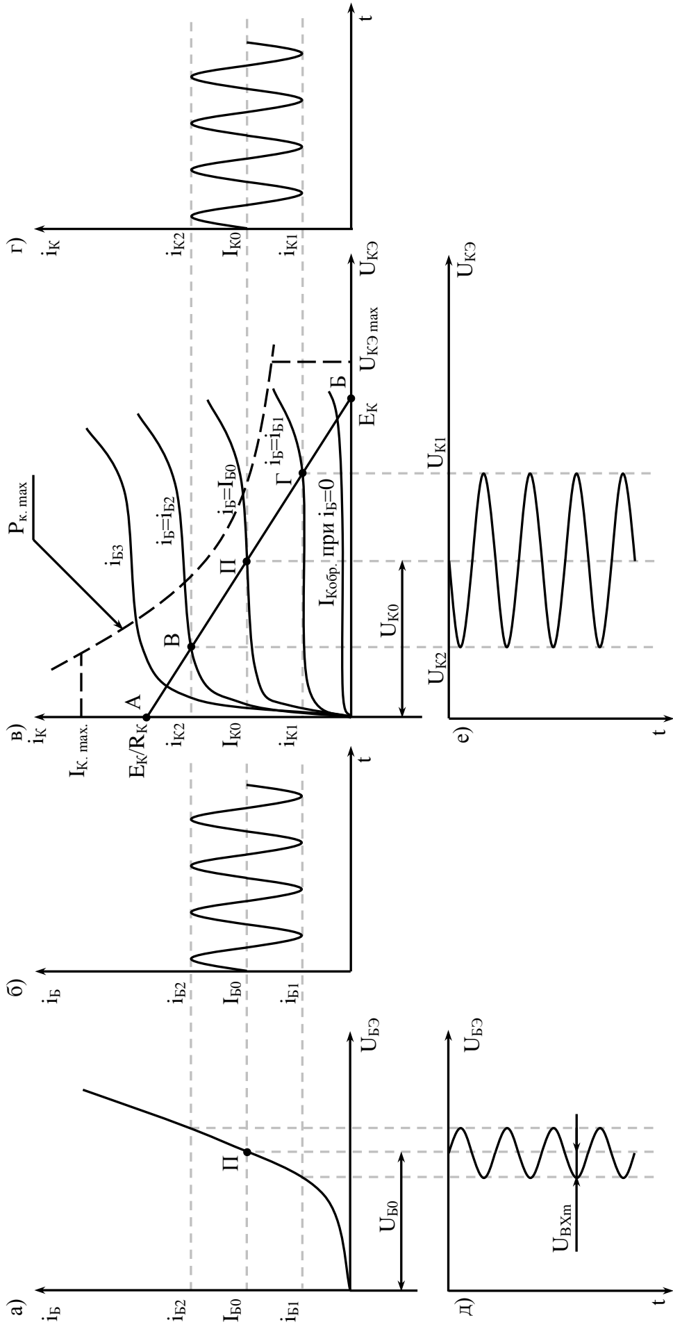
Рис. 1. Характеристики транзистора и графики напряжений и токов: а) входная характеристика б) ток базы в) выходные характеристики г) ток коллектора д) напряжение базы е) напряжение коллектора
